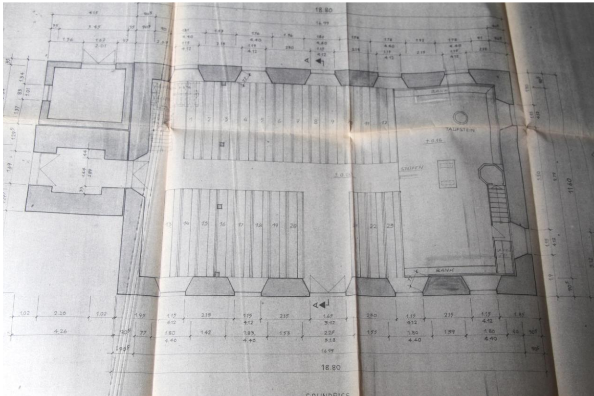
Grundriss der in 1881 erbauten Kirche
