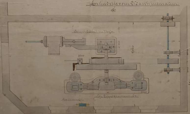
Grundriss vom Wassermaschinenraum
