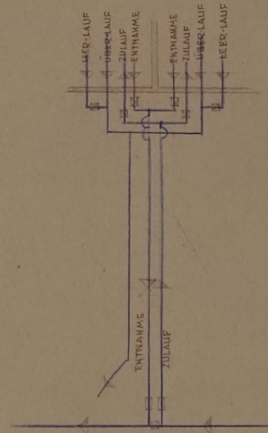
• LEITUNGS-SCHEMA •
