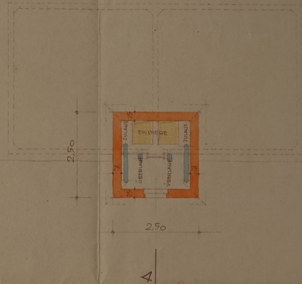
• GRUNDRISS II-II •
