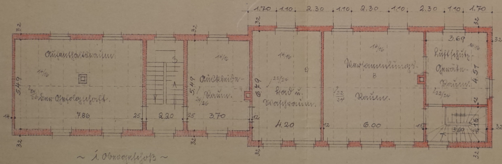
~ 1. Obergeschoss ~
