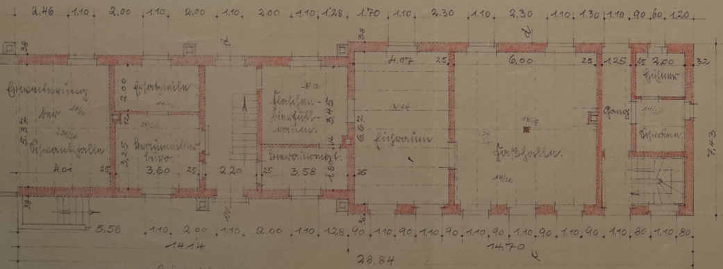
~ 2. Obergeschoss ~
