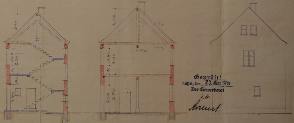
~ Schnitt n-s ~
