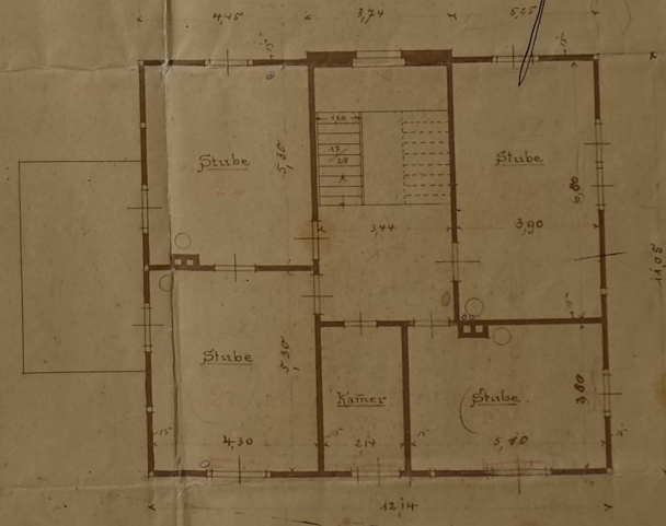
I. Obergeschoss.
