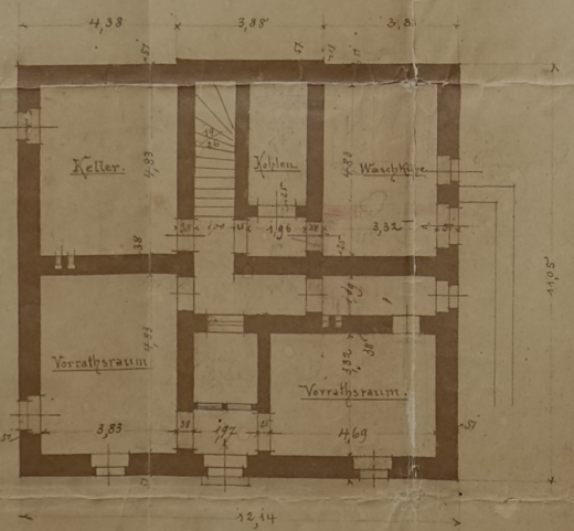
Kellergeschoss.
