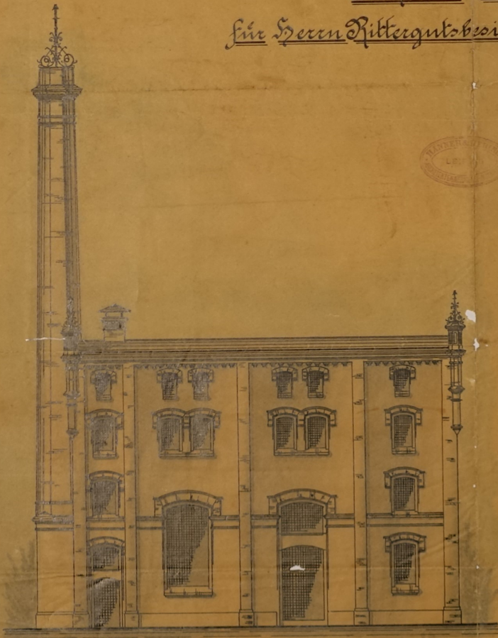
Ansicht.
