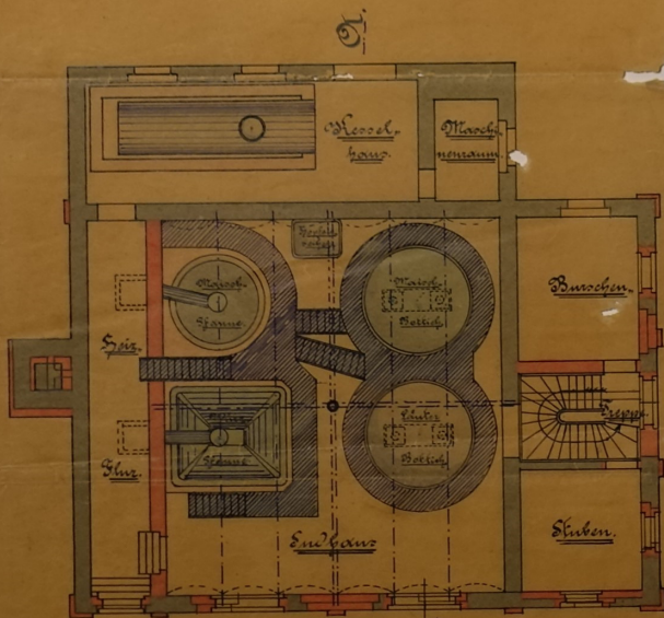
Grundriss I.
