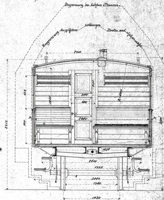
Schnitt A-B.
