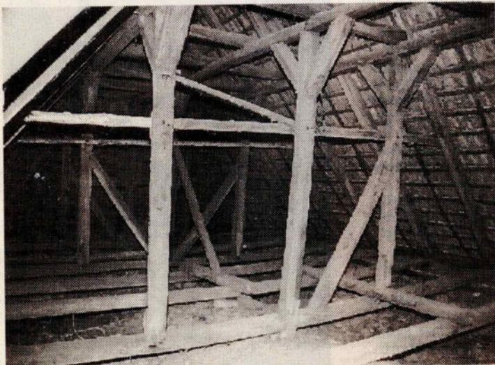
Gefährliche Schiefelage des Dachgebälks im Chorbereich der Kirche. Die Konstruktion hat sich im ganzen bereits um etwa 15 Grad in Richtung des Kirchschiffs geneigt.
